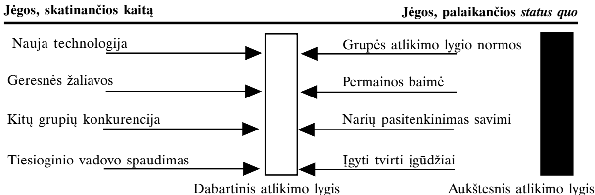
1 pav. Jėgų lauko diagrama
